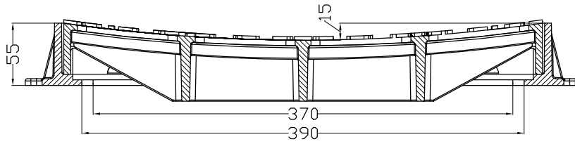
SEZIONE A-A
