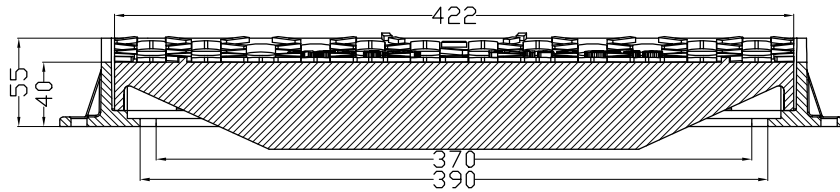
SEZIONE B-B
